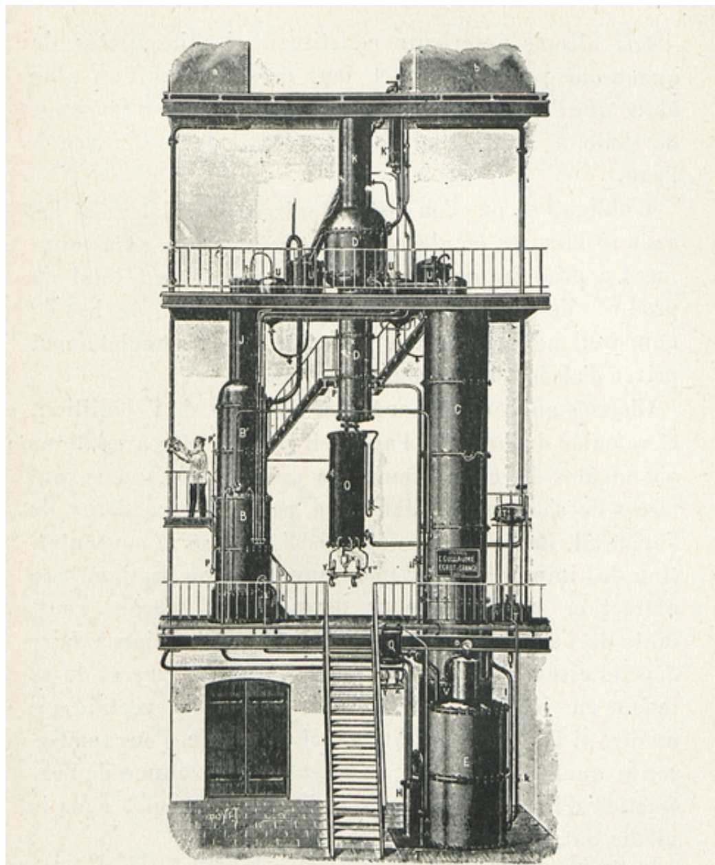
FIG. 83. — Appareil de rectification continue (système Guillaume).
