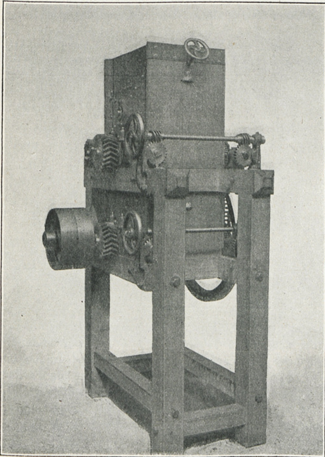
FIG. 46. — Broyeur de féculle verte.
