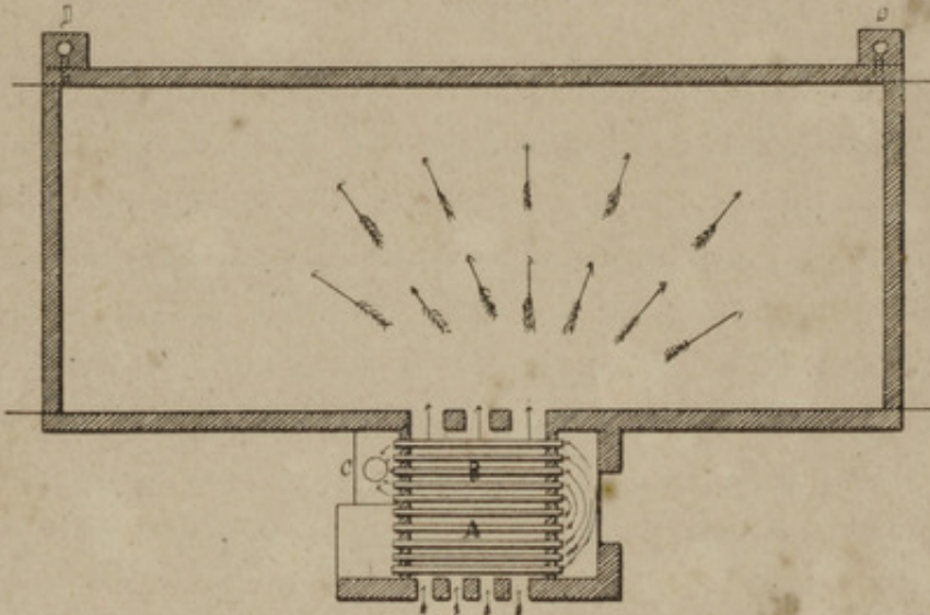
Fig. 1. — Plan de la substruction et du foyer.
