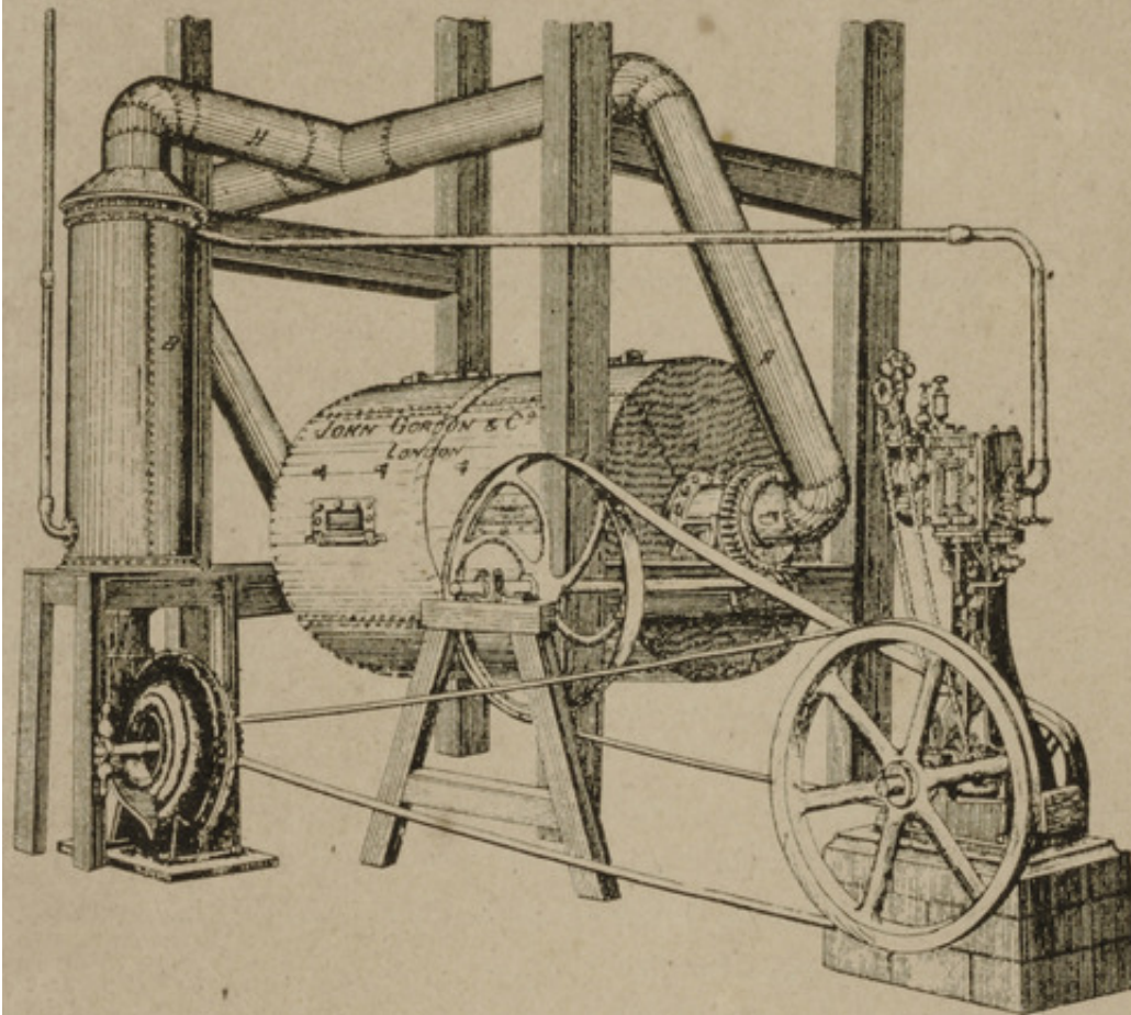
Fig. 1. — Séchoir de Guardiola.
