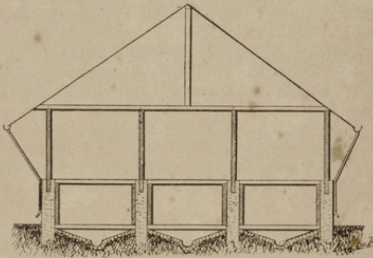
Fig. 2. — Élévation transversale.
