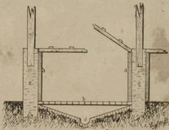
Fig. 3. — Détail d'un bac : a, revêtement en bois ; b, fond percé du bac ; c, murette de réparation ; d, rigole d'écouement.
