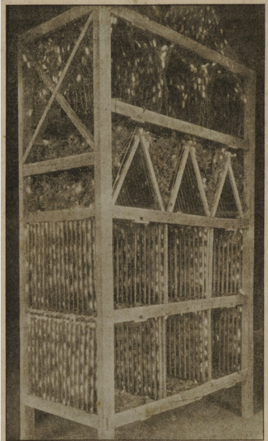
Vue d'ensemble d'un bâti comprenant des claies cocoonnières Davril, un étage de claies cocoonnières prismatiques de Nanisana et trois arceaux en bruyères représentant l'encabanage le plus communément employé.
